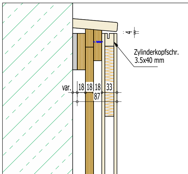
Maßst. 1:5
